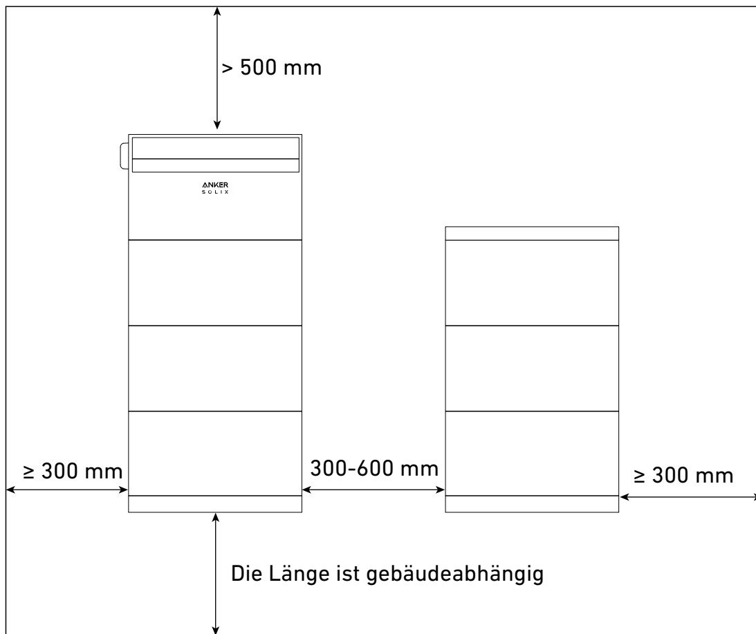
Abbildung: Installationsraum für wandmontierte Module.
