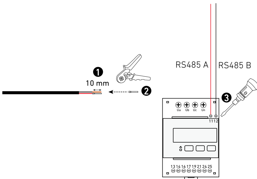
PV-seitiger Stromsensor
