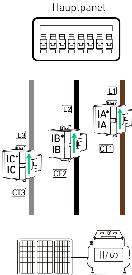
Bestands-PV-System
