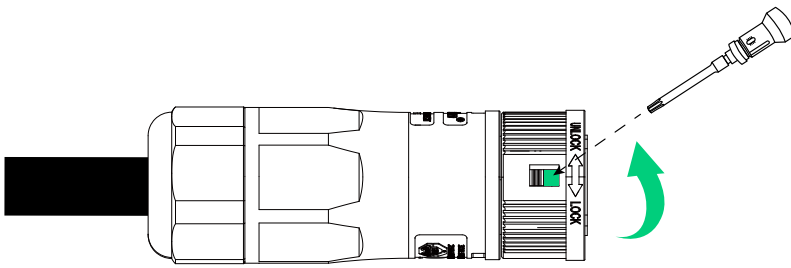
Abbildung: Entfernen Sie die Wechselstrom-Stecker.
